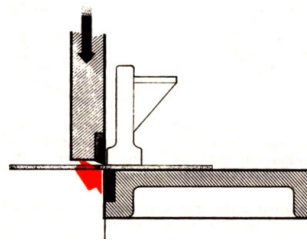
Couteaux
