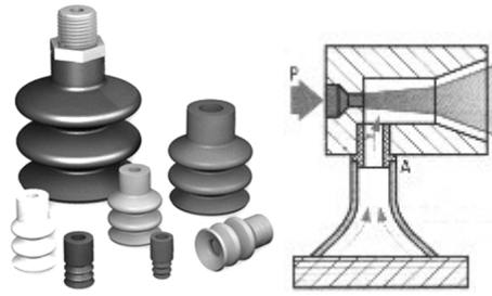
ventouse
