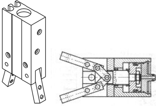
Pincés
